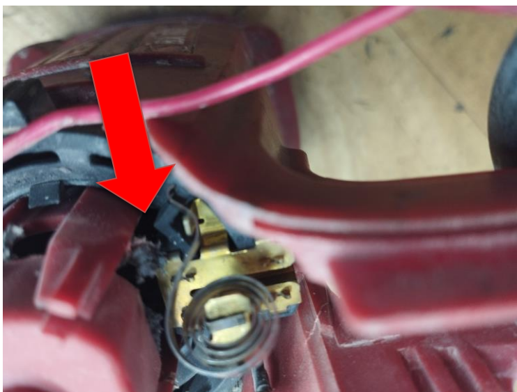
Obr.3 Poškodenie držiaka uhlíkov
