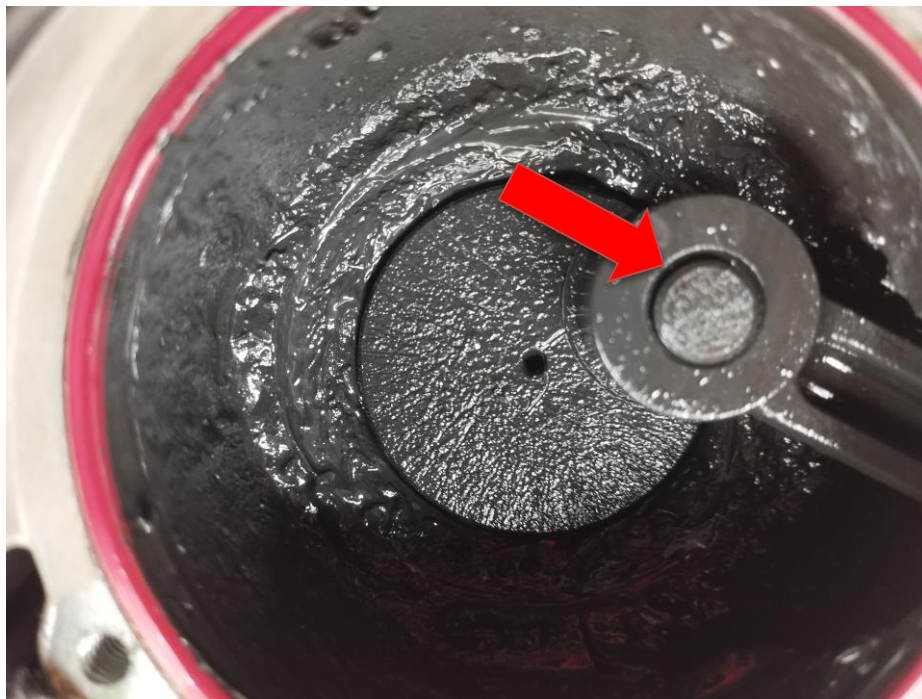
Obr.4 Zväčšená vôľa ojnice
