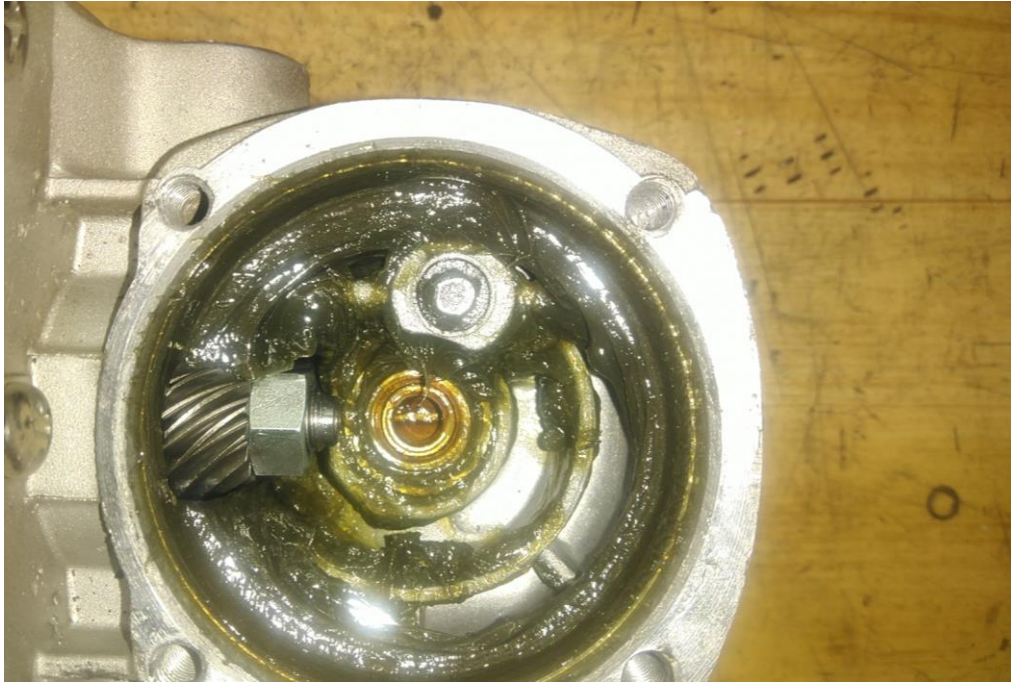
Obr.1 Poškodenie aretačného kolíka
