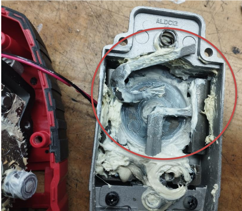
Obr.1 Poškodenie hnacieho mechanizmu
